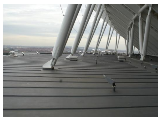
Wembley EP-PV F 1,5 mm Ral 7012 Lepljen sistem s Flexocol A89
